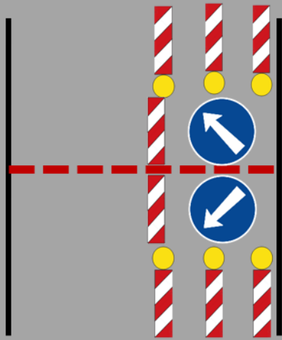
Překop komunikace po polovinách
